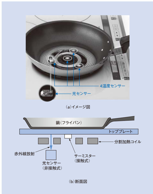
図4 | 光センサーと4個の温度センサー 鍋温度を直接測定する光センサーと、4個の温度センサーで、鍋温度をきめ細かく制御するとともに鍋の空だきなどを防止する。
