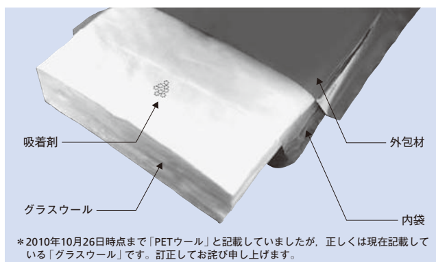
図11 | フレックス真空断熱材 貯湯タンクの断熱材にフレックス真空断熱材を採用し、断熱性能を向上させた。
