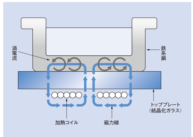
図3 | IHの加熱原理 磁力線が鍋底を通ると、鍋底に磁力線を打ち消す方向に渦電流が発生し、鍋の電気抵抗R、渦電流Iによるジュール熱( I^2R )によって、鍋自体が発熱する。
