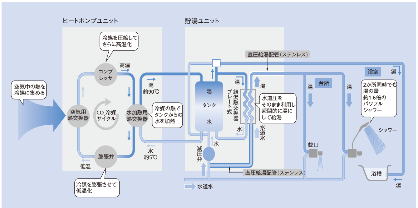
図12 | 水道直圧給湯方式エコキュートのシステム構成イメージ リモコンのボタン操作によってふろ自動運転を行うことができるフルオートタイプの水道直圧給湯方式エコキュートのシステム構成のイメージを示す。
