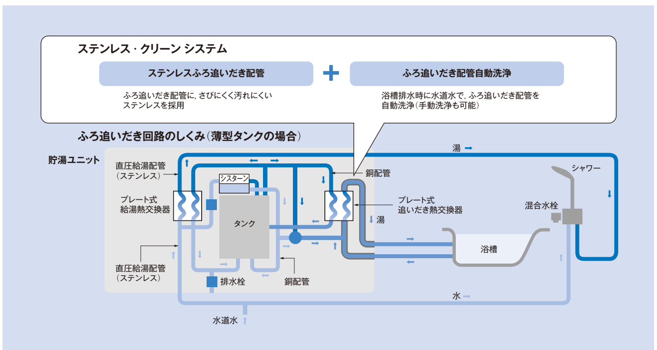
図13 | ステンレス・クリーンシステムのイメージ 配管にステンレスを採用し、配管内を自動洗浄する機能を搭載することで、配管内を清潔に保つ「ステンレス・クリーンシステム」の概要を示す。
