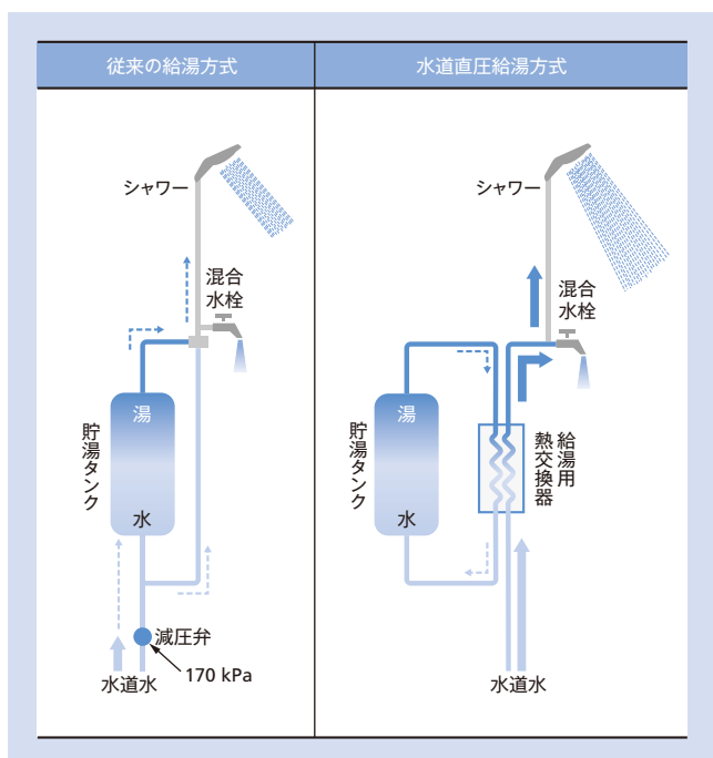
図9 | 従来の給湯方式と水道直圧給湯方式の比較 水道直圧給湯方式は、減圧弁およびタンク内を經由しないで加熱給湯するため給水圧力に近い給湯圧力を確保できる。
