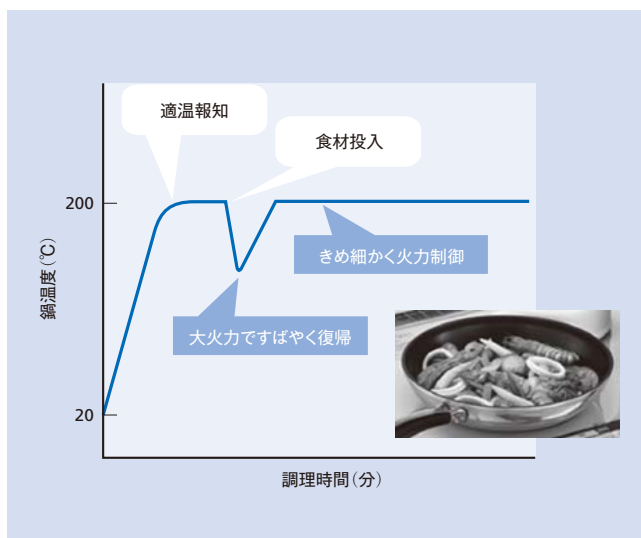
図5 | 適温調理の200°C温度制御例 調理の失敗をなくするため、コツとなる「火加減」を「温度加減」に置き換えた。
