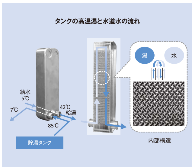
図10 | 給湯熱交換器による水道水の加熱構造 給湯熱交換器には、コンパクトで伝熱面積が大きい高性能プレート式熱交換器を採用している。
