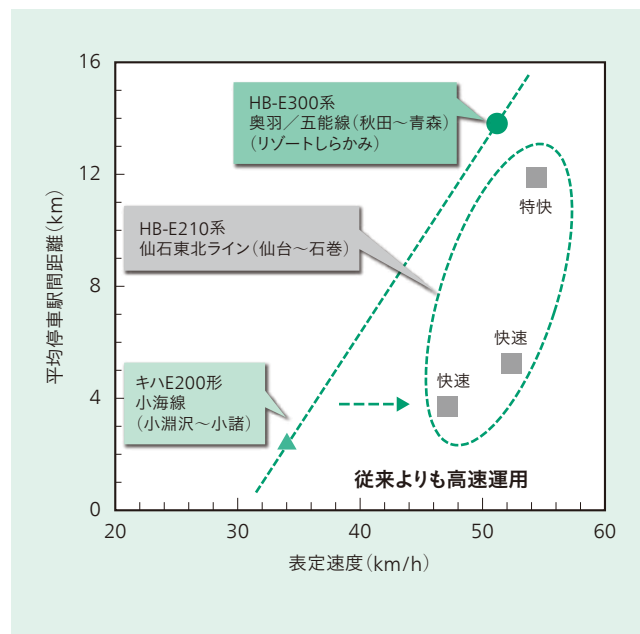
図7 ハイブリッド車両の運用形態の比較
