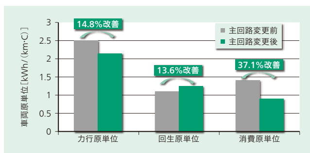
図8 近郊および通勤路線による省エネルギー効果の検証 従来システムと比較し、約40%の車両原単位低減を確認した。
