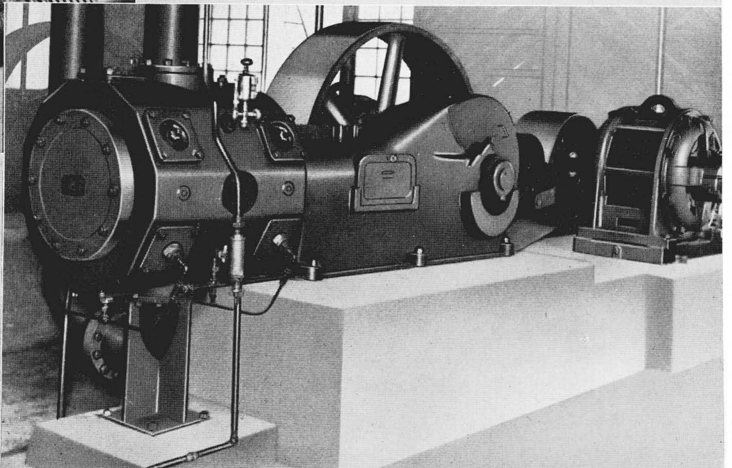
100 HP 横型一段複動空気圧縮機
