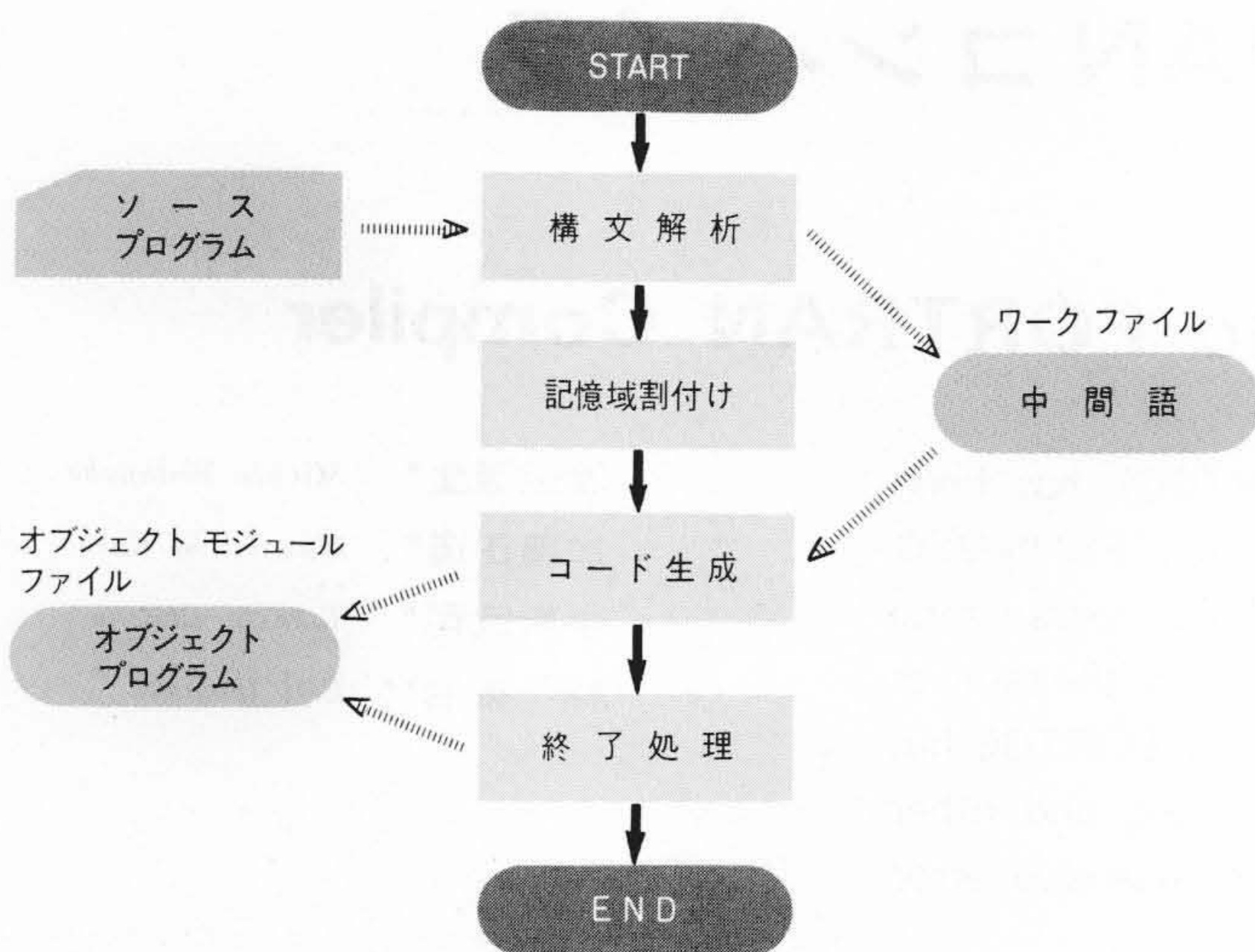
図1 通常のFORTRANコンパイラにおける処理の流れ 通常のFORTRANコンパイラでは、マルチパスになっていて、その間にワークファイルとの入出力が行なわれる。
