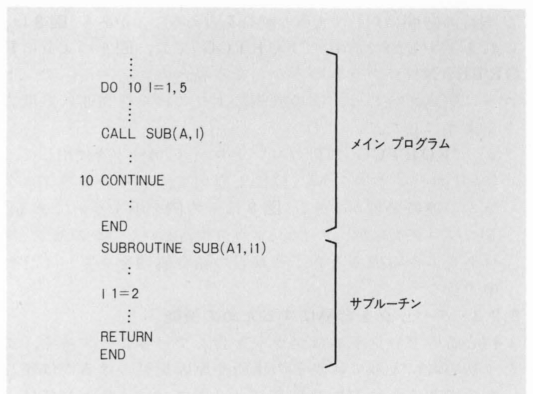
図9 DOパラメータを変更している例 DOループの制御変数がサブルーチンSUBの中で変更されている。
