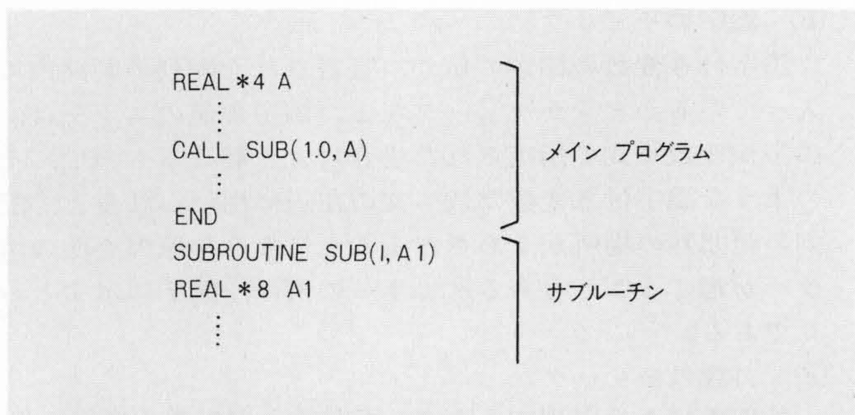
図8 引数が一致しない例 実引数と仮引数とは、個数、順序、種類、形及び長さが一致しなければならない。
