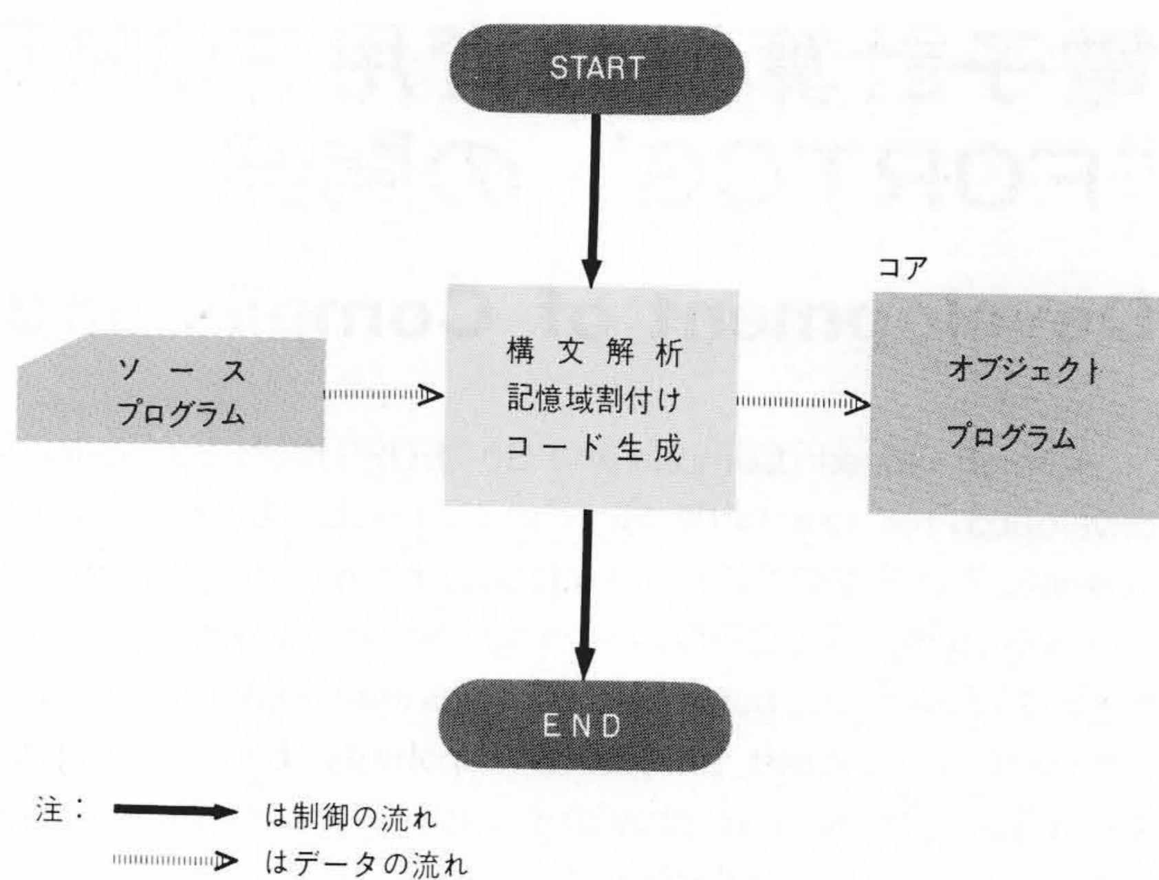
図2 “FORTCG”における処理の流れ “FORTCG”では1パスでワークファイルとの入出力も行なわれず、オブジェクトプログラムは直接実行可能な形でコア上に作成される。
