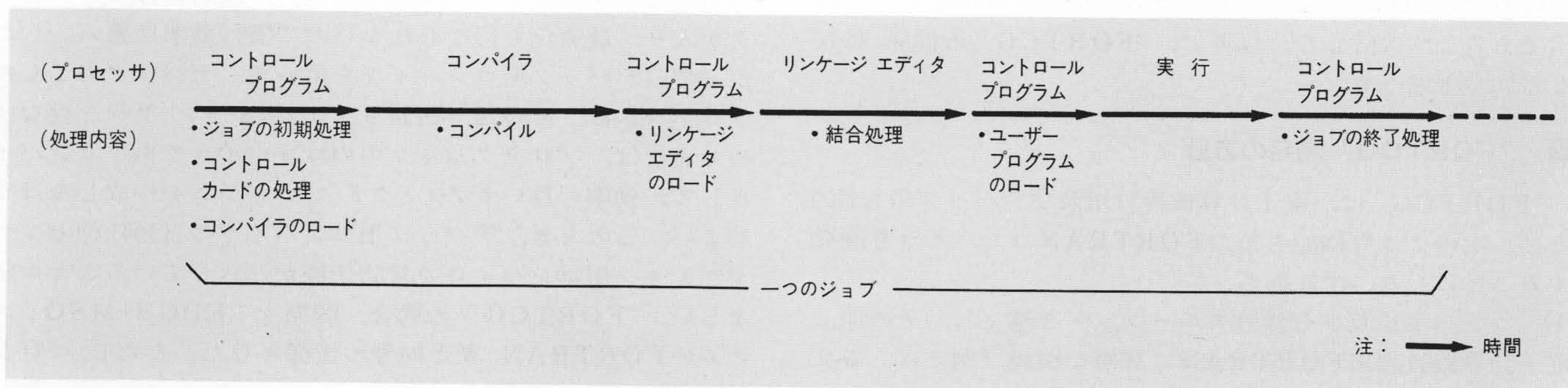
図3 通常のシステムにおける処理の時間経過 通常のシステムでは、コントロールプログラム、リンケージエディタのオーバヘッドが大きい。
