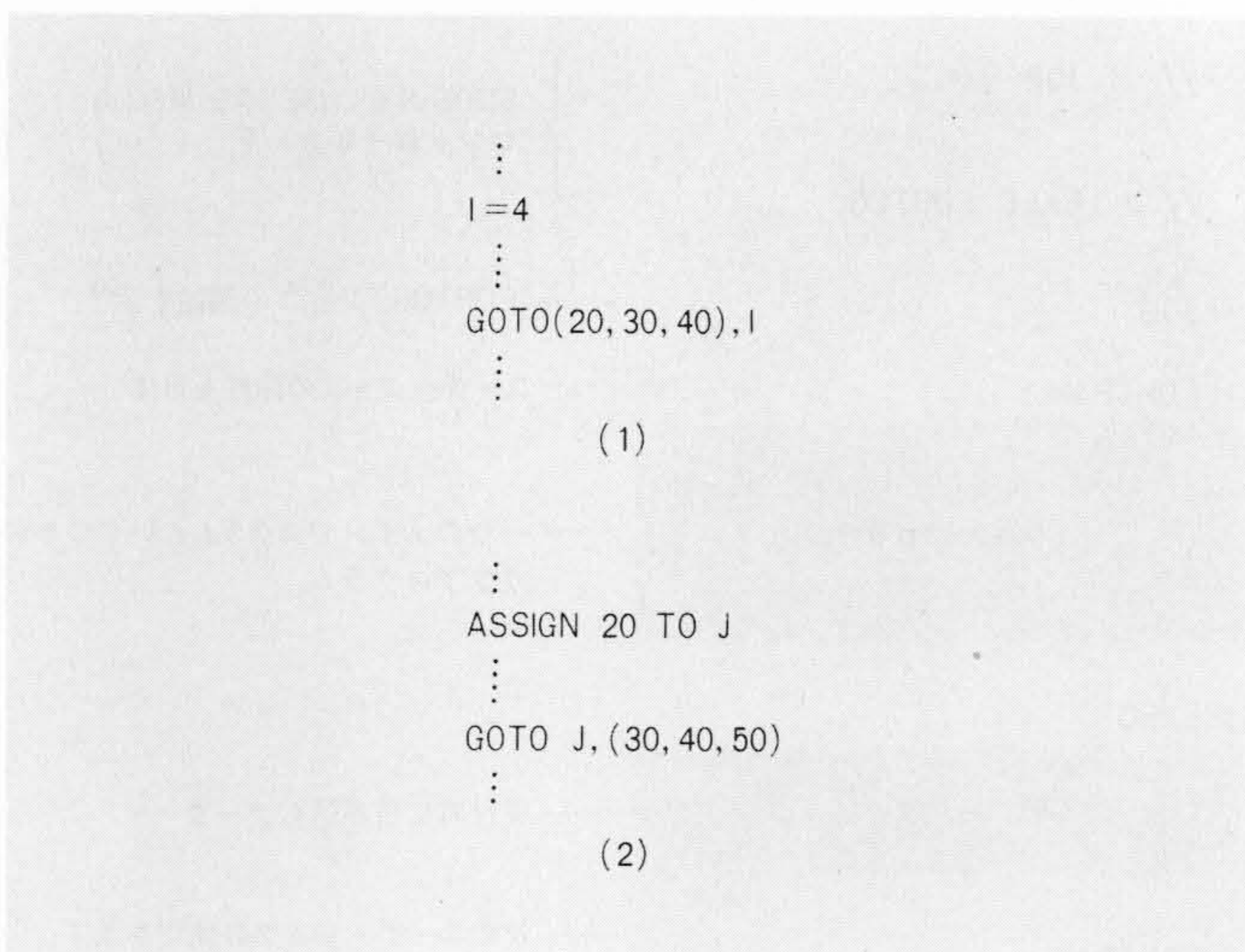
図6 飛び先の誤り例 計算形GOTO文、割当て形GOTO文でIあるいはJがそれぞれ範囲内に入っていない。いずれの場合も次の文が飛び先となる。
