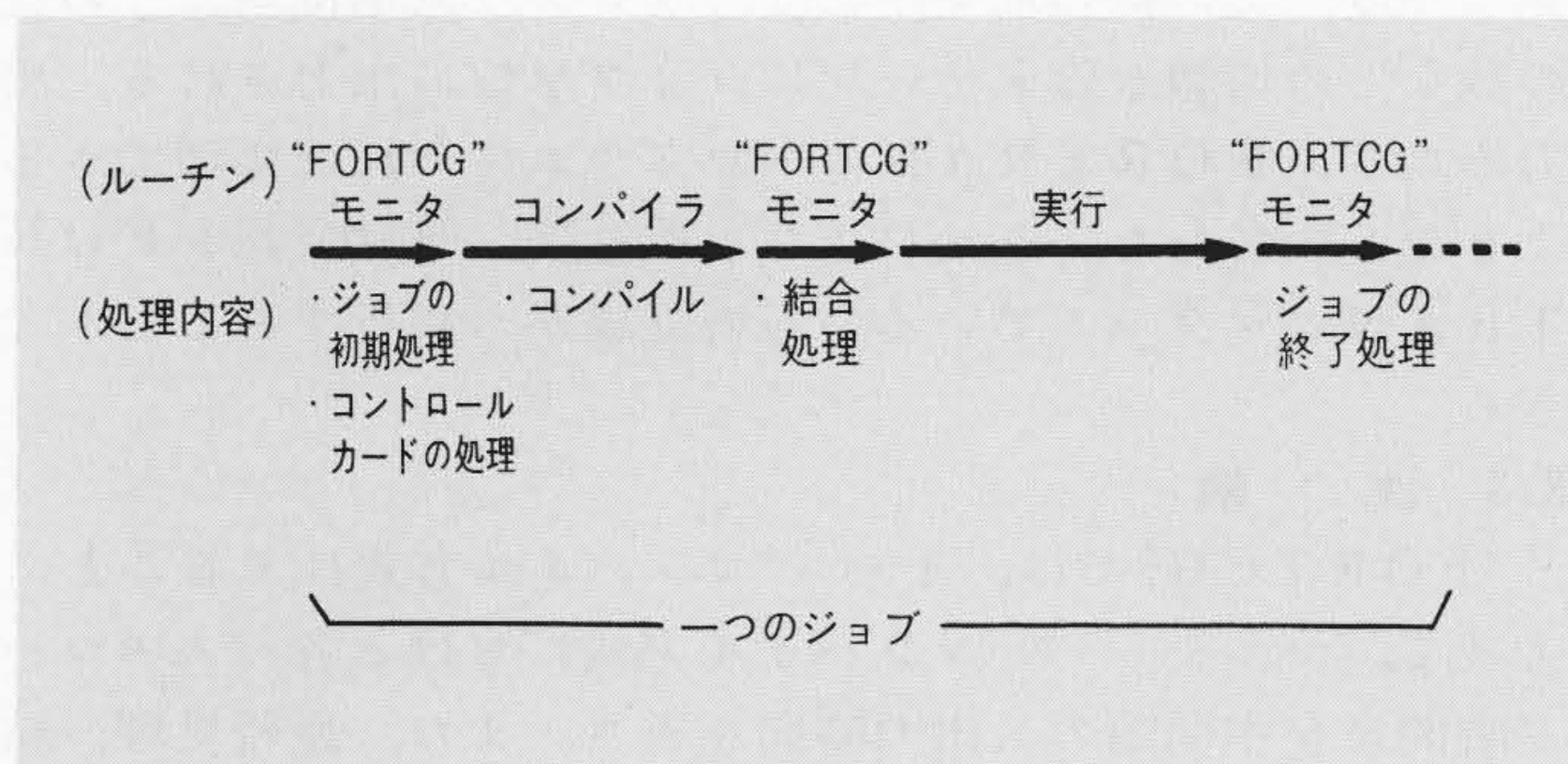
図4 “FORTCG”における処理の時間経過 “FORTCG”では、連続処理、結合処理をコンパイラの中のコントロールルーチンで行なう。
