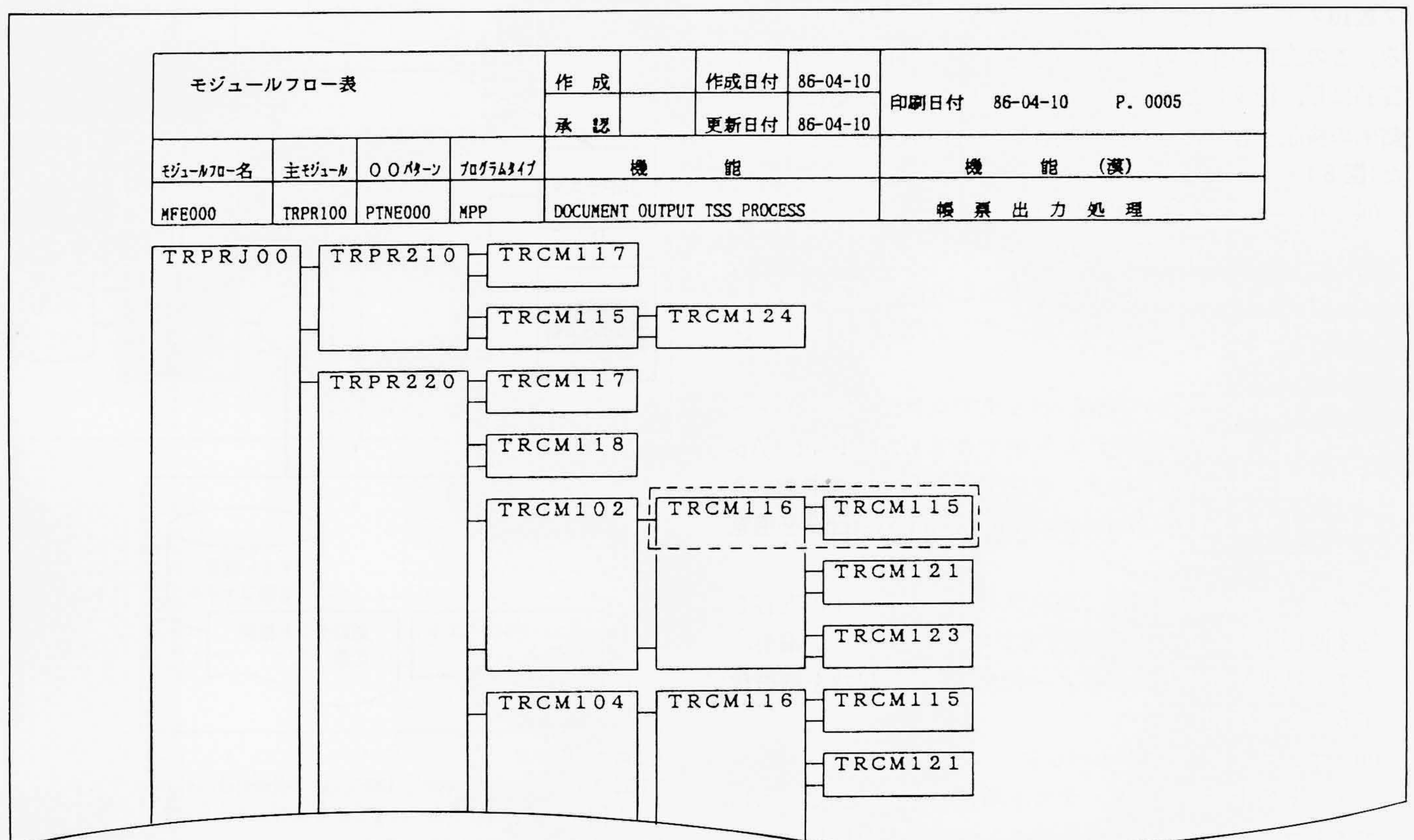
図4 トランザクション定義支援によるモジュールフロー出力例 自動清書機能により、設計時の試行錯誤作業を支援する。
