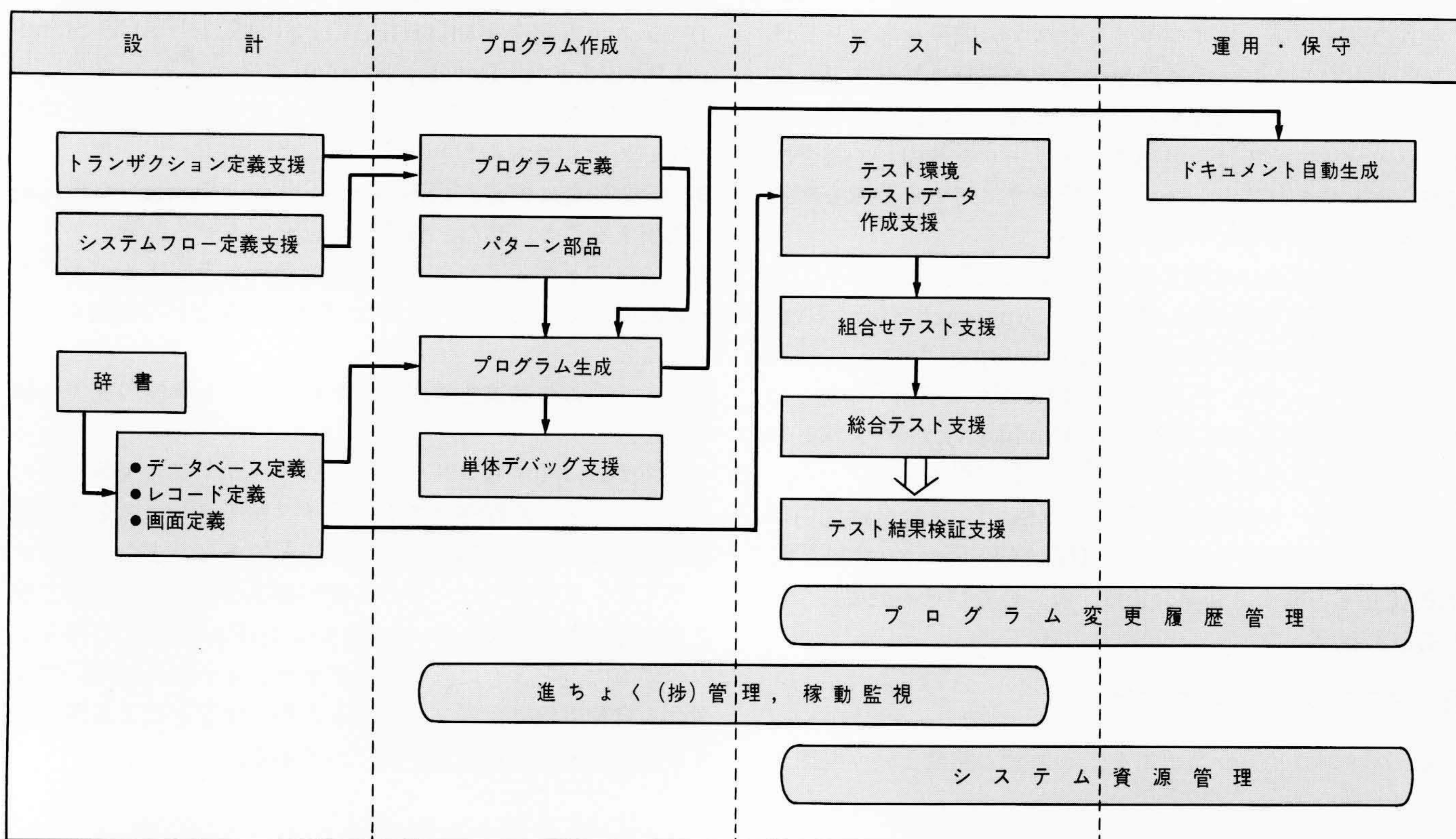
図2 HIPACE-Financial 開発支援ツールのサブシステム構成 各工程の作業を支援し、各工程での成果物が次工程の入力となる。
