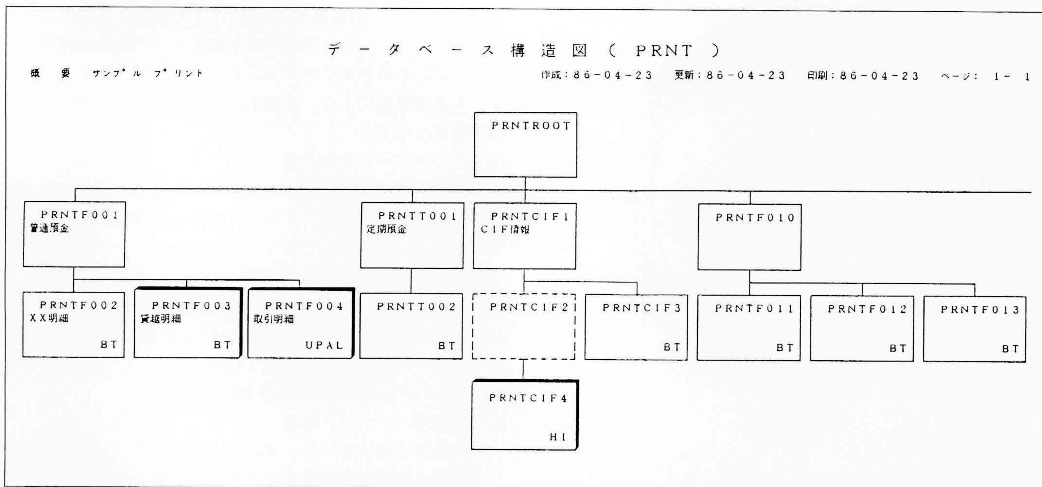
図5 データベース定義支援によるデータベース構造図の出力例 セグメントの構造をイメージとして把握できる。
