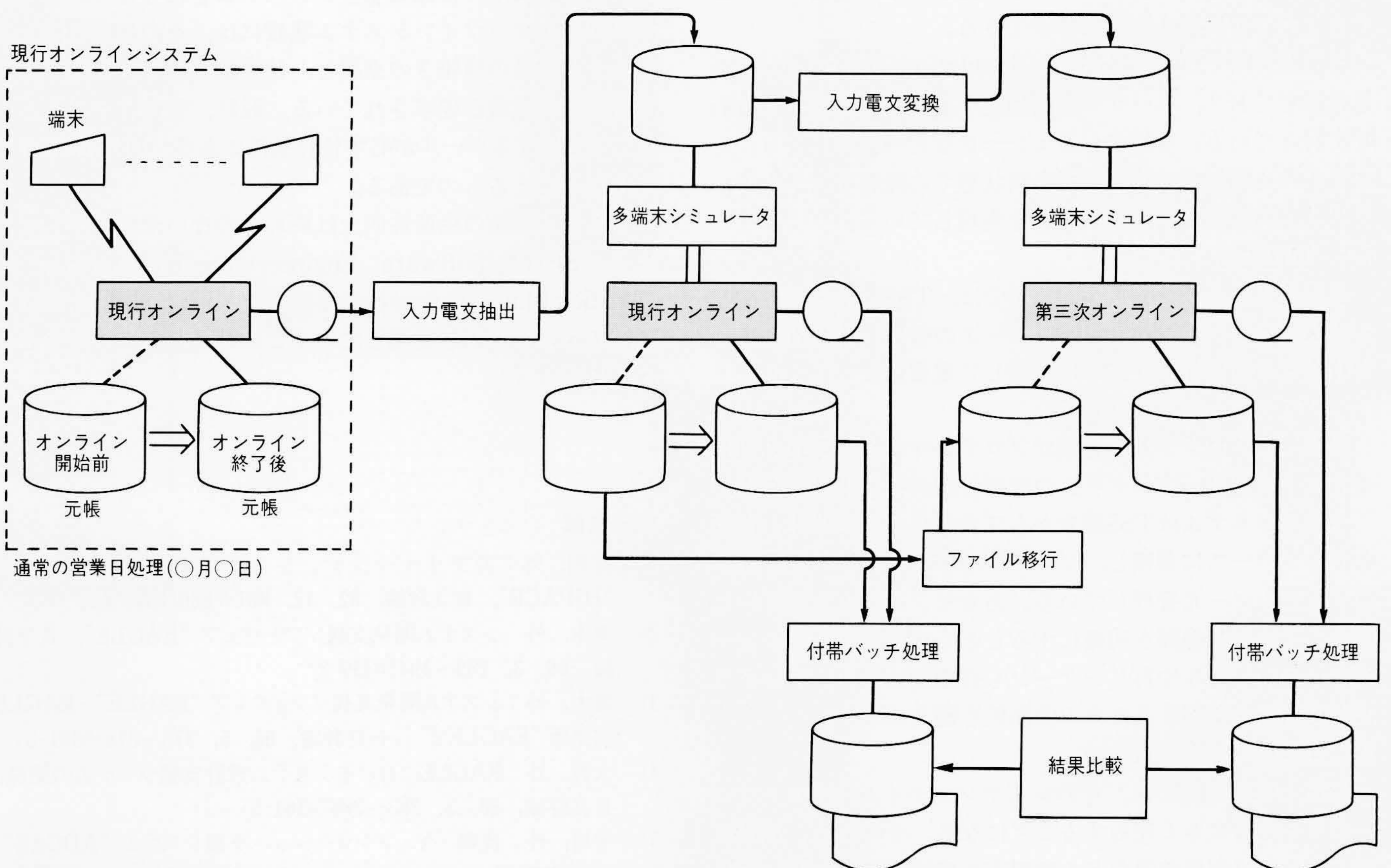
図 8 並行ラン確認テストの概要 現行システムと同一の処理を新システムで行い、両者の処理結果を比較する。
