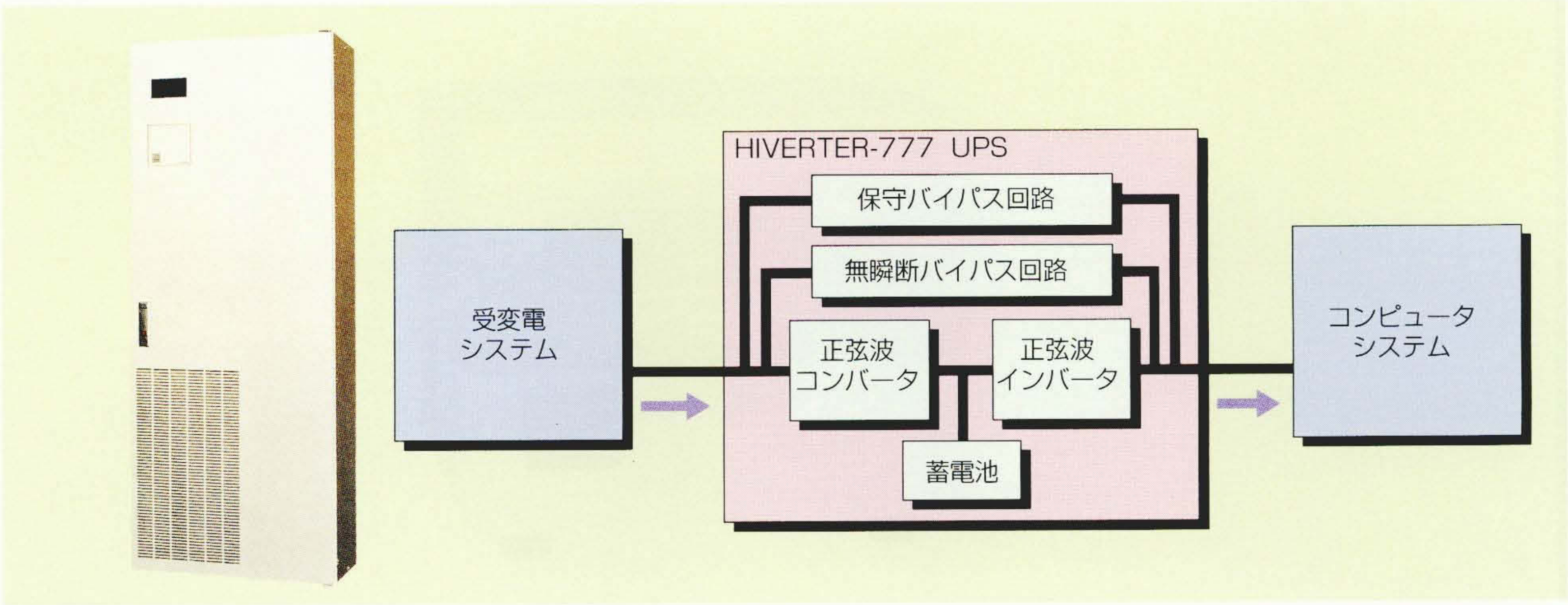
無停電電源装置「HIVERTER-777シリーズ」の外観およびシステム構成
