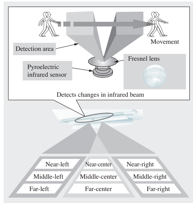
Fig. 2—Eco-sensor.
